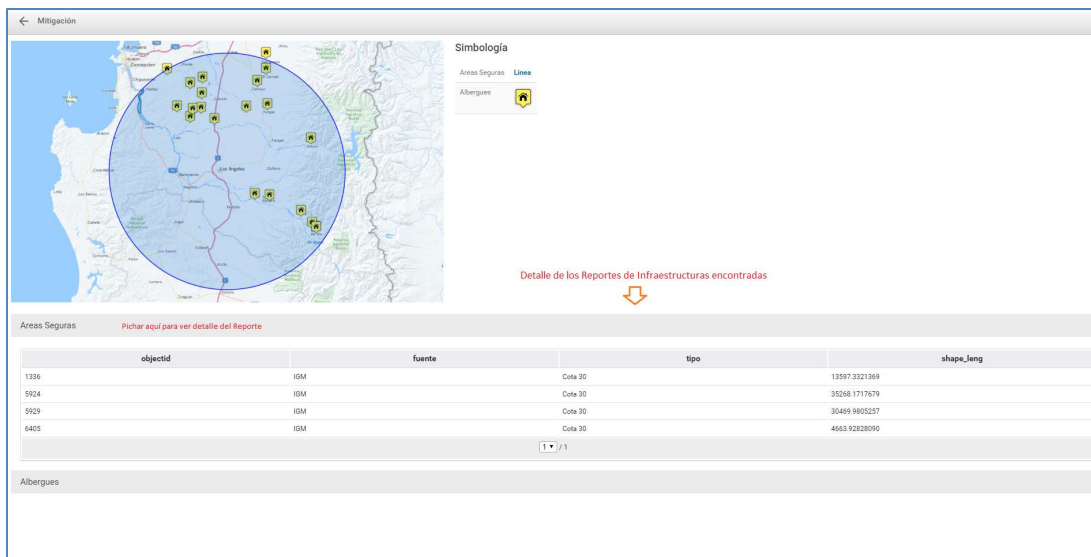
Figura 75: Reporte Mitigación
