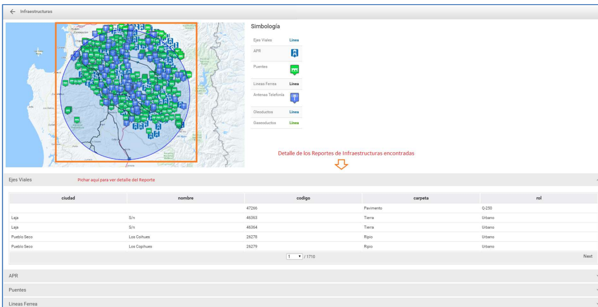
Figura 73: Reporte Infraestructuras
