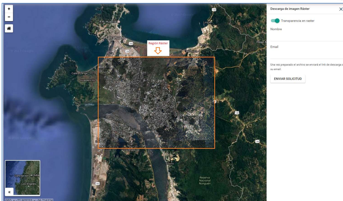
Figura 23: Región Ráster
