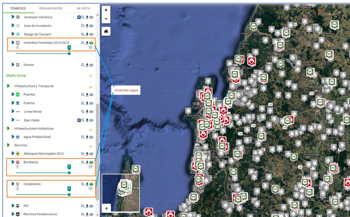
Figura 36: Encender capas
